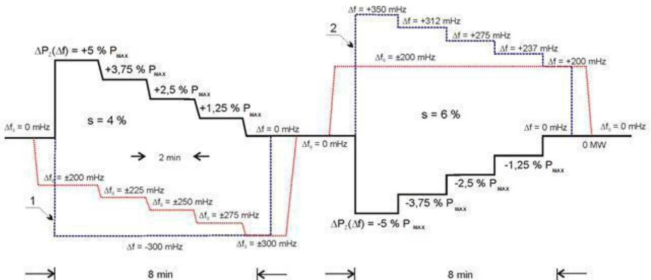
Rys. 4 Sprawdzenie odpowiedzi częstotliwościowej przy zmianach: strefy niezułości odpowiedzi częstotliwościowej, statyzmu oraz odchyłki częstotliwości
